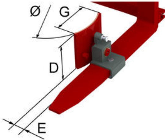
套装式夹臂 - 机械式旋转
