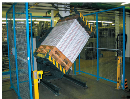
固定式转换装置 T451W/099 (Stationary MH Equipment)
